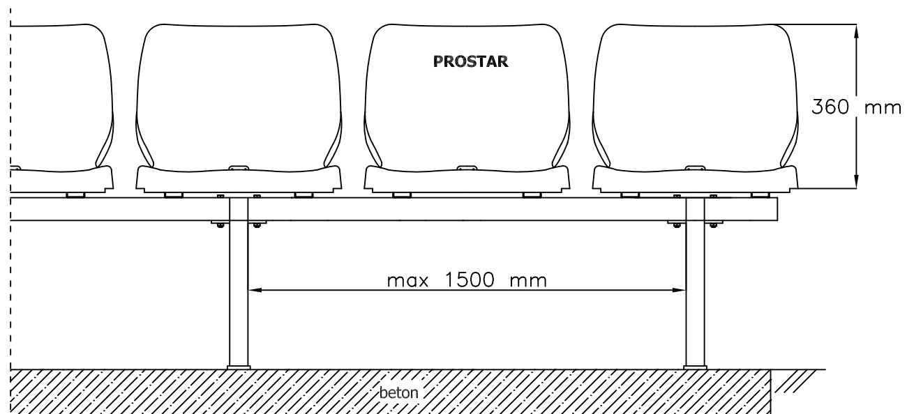
POHL'AD SPREDU
