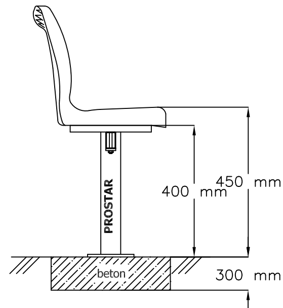
POHL'AD ZBOKU
